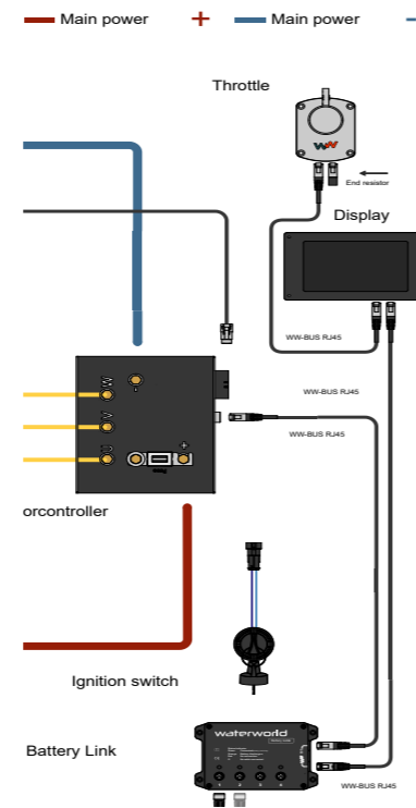
Voorbeeld aansluitschema
